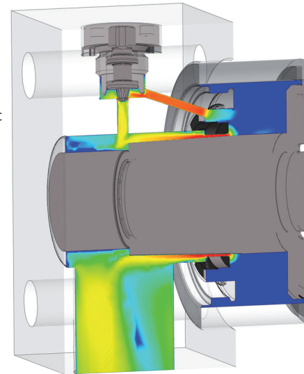
Vitesse d'écoulement
