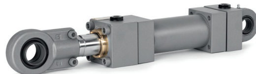
CH ISO 6020-2/3
