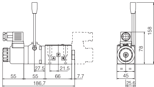
DHL-06*/MV 质量: 2.4kg(单电磁铁) DHL-07*/MV (虚线) 质量: 2.7kg(双电磁铁)
