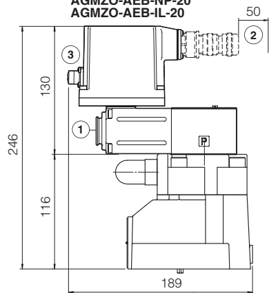
AGMZO-AEB-NP-20 AGMZO-AEB-IL-20
