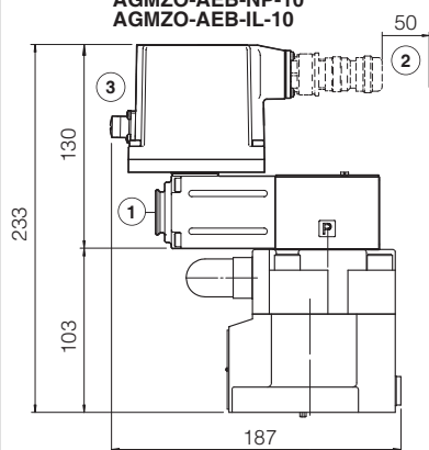
AGMZO-AEB-NP-10 AGMZO-AEB-IL-10
