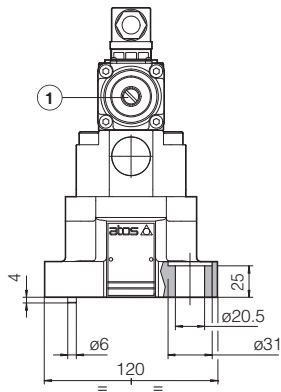
AGMZO-A-32
