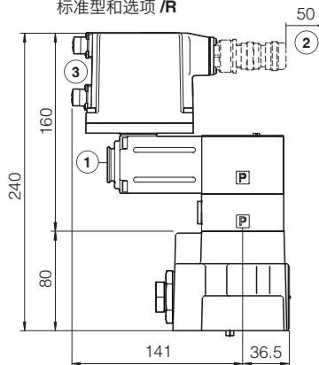
AGRCZO-AES-BC-10 AGRCZO-AES-BP-10 标准型和选项 /R
