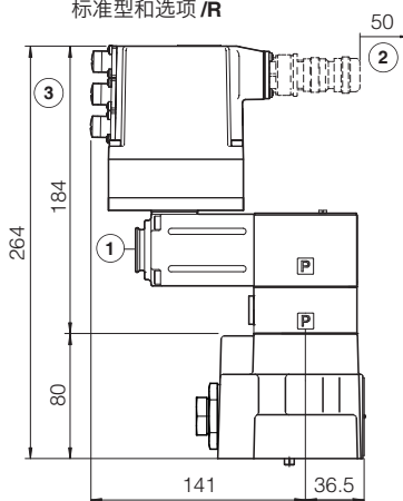
AGRCZO-AES-EH-10 标准型和选项 /R
