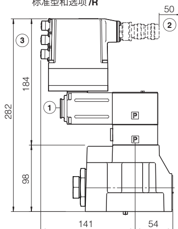
AGRCZO-AES-EH-20 标准型和选项 /R
