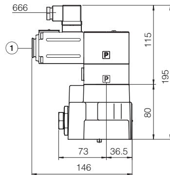
AGRCZO-A-10 标准型和选项/R
