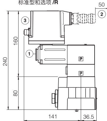
AGRCZO-AEB-NP-10 AGRCZO-AEB-IL-10 标准型和选项 /R
