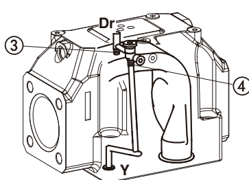
泄油路结构
