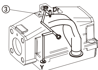
泄油路结构
