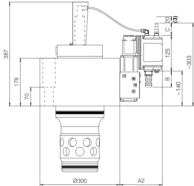
LIQZP-LEB-*-1002 LIQZP-LES-*-1002
