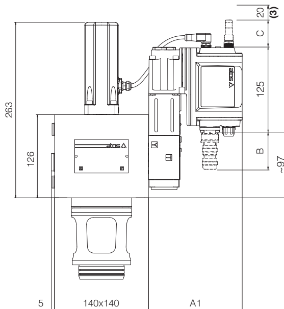
LIQZH-LEB-632 LIQZH-LES-632
