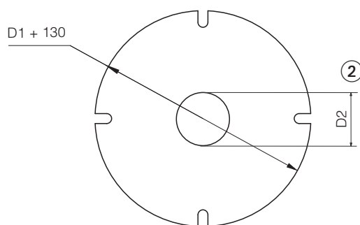
Vista superiore telo protettivo
