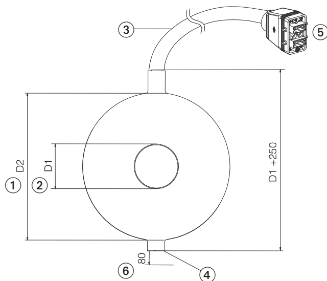
Vista superiore coperta MHB
