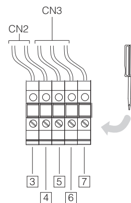
Collegamenti cancello di sicurezza e termocoppia
