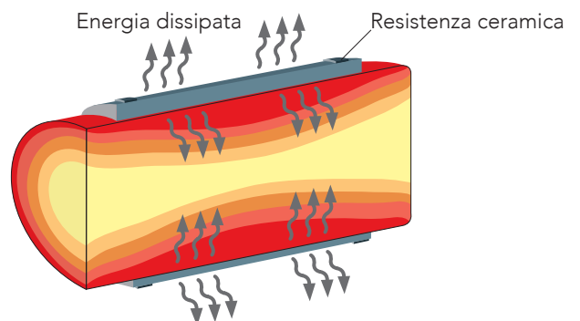
Calore trasmesso per conduzione
