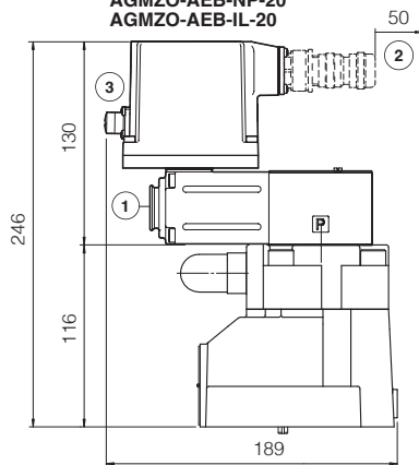
AGMZO-AEB-NP-20 AGMZO-AEB-IL-20
