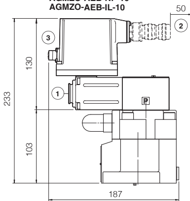
AGMZO-AEB-NP-10 AGMZO-AEB-IL-10
